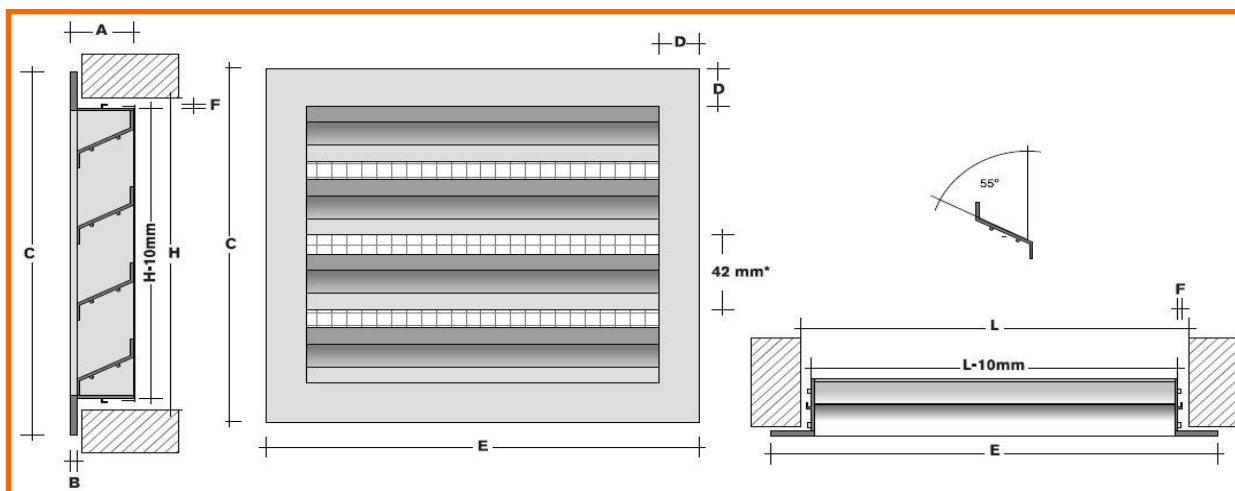
GAE - Grelha de Ar Exterior - Dimensões
